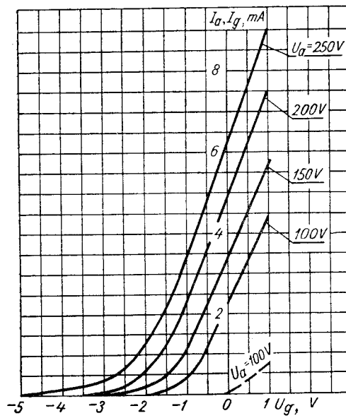
I_a, I_{gT} = f(U_{gT}) (каждого триода) (for each triode)
