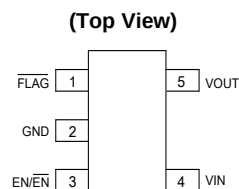
SOT-23-5
