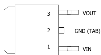
TO-252 3L
