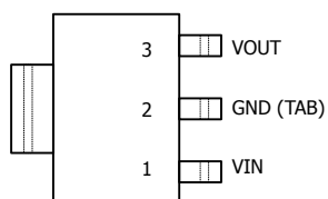
SOT-223
