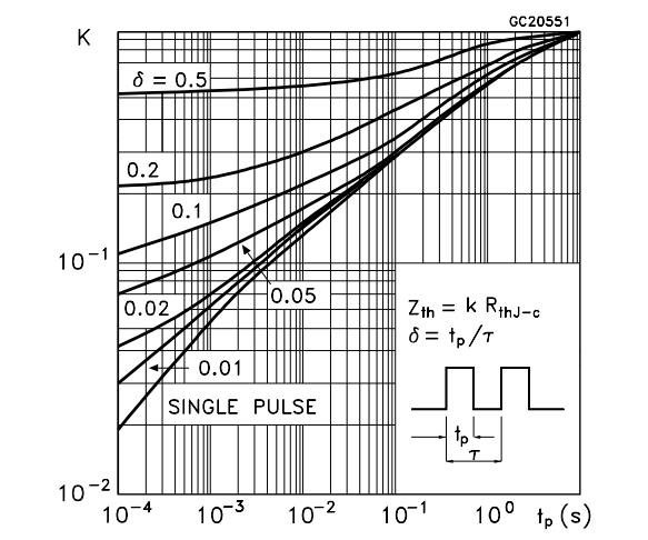
Thermal Impedance
