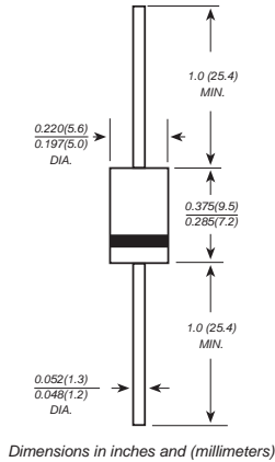
DO-201AD
