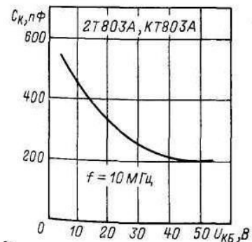
Зависимость емкости коллекторного перехода от напряжения коллектор-база
