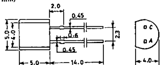
外形図 3000B-S2TR (unit: mm)
