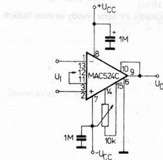
Informativní zapojení nulování výstupního zbytkového napětí
