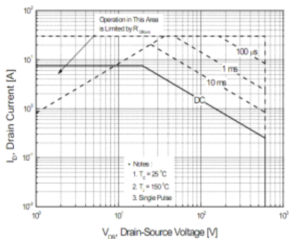
图 6-1 SIF7N60D(TO-220)
