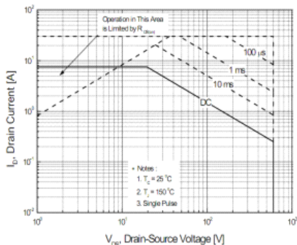
图 6-2 SIF7N60D(TO-220FP)
