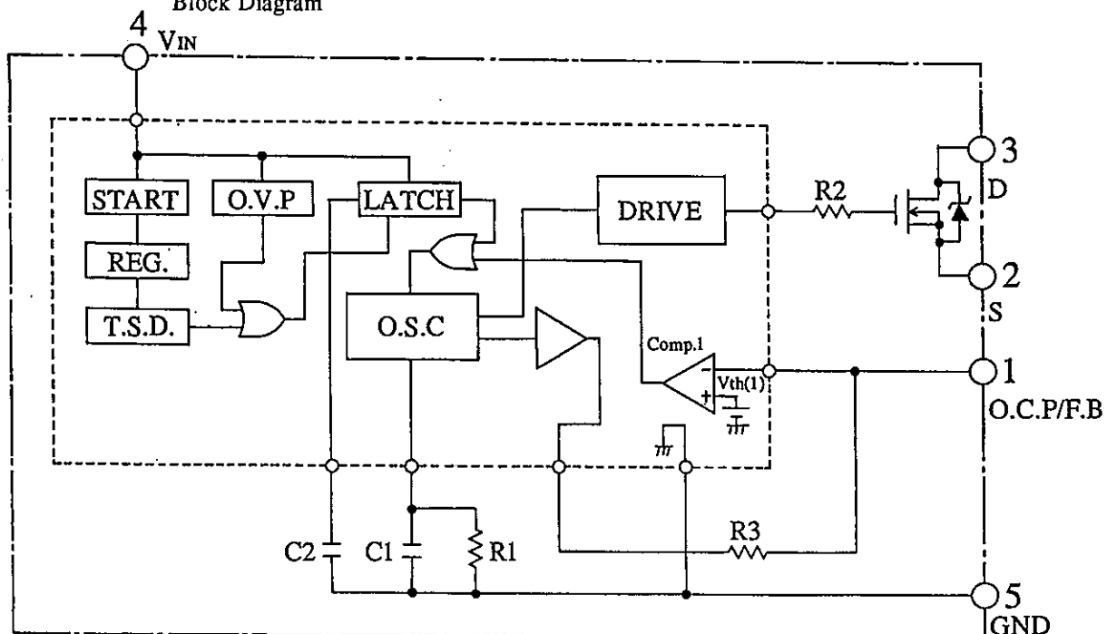
各端子機能 Function of Terminal
