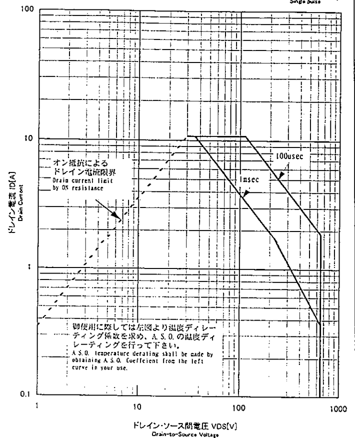
STR-F6552 MOS FET A.S.O:曲線 curve
