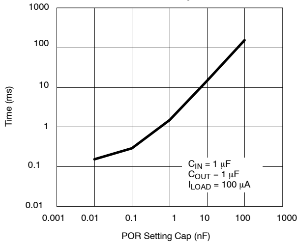
POR Delay
