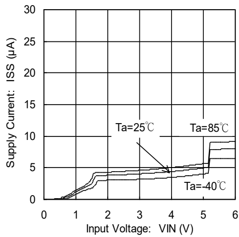
XC6116, XC6117(5.0V)
