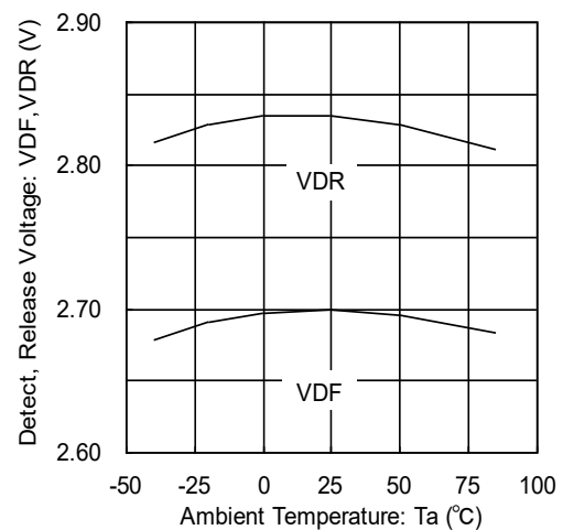
XC61X1~XC61X7 (2.7V)
