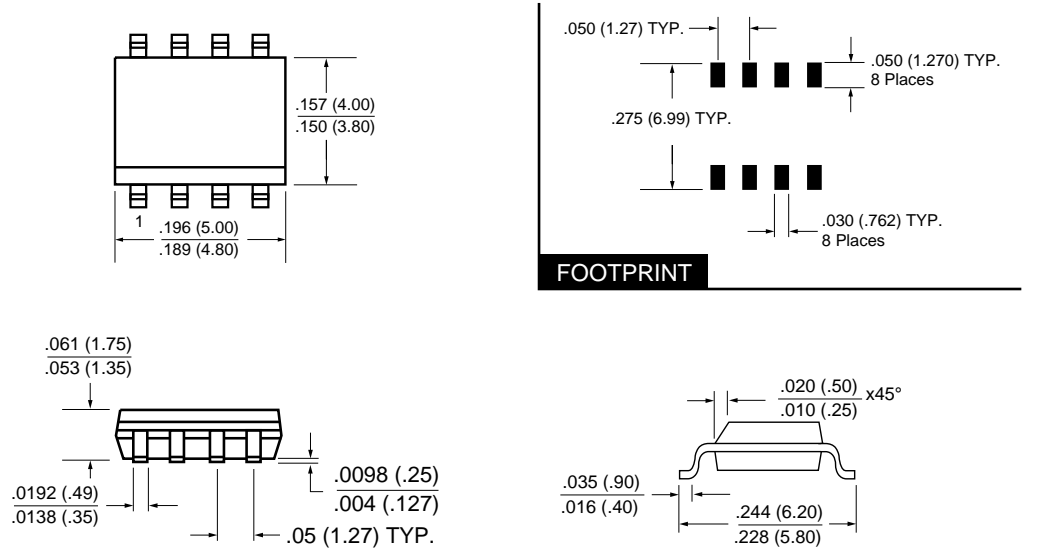
8pn JEDEC SOIC ILL.1
